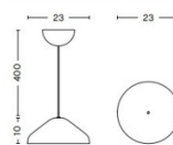
Pao Steel Pendant 230
